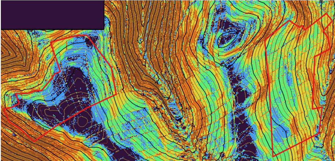
Abbildung 2: Hangneigung (dunkelblau: < 3°, hellblau: < 5°, grün: < 7°, gelb: < 10°, orange: < 15°, rot: >= 15°) sowie Höhenlinien (dargestellt in Schwarz, 10 m Höhenunterschiede) und Grenzen des Solarparks. Die Darstellung basiert auf eigenen Berechnungen, aufbauend auf dem DGM1. Datenquelle: Landesamt für Digitalisierung, Breitband (Bayern)
